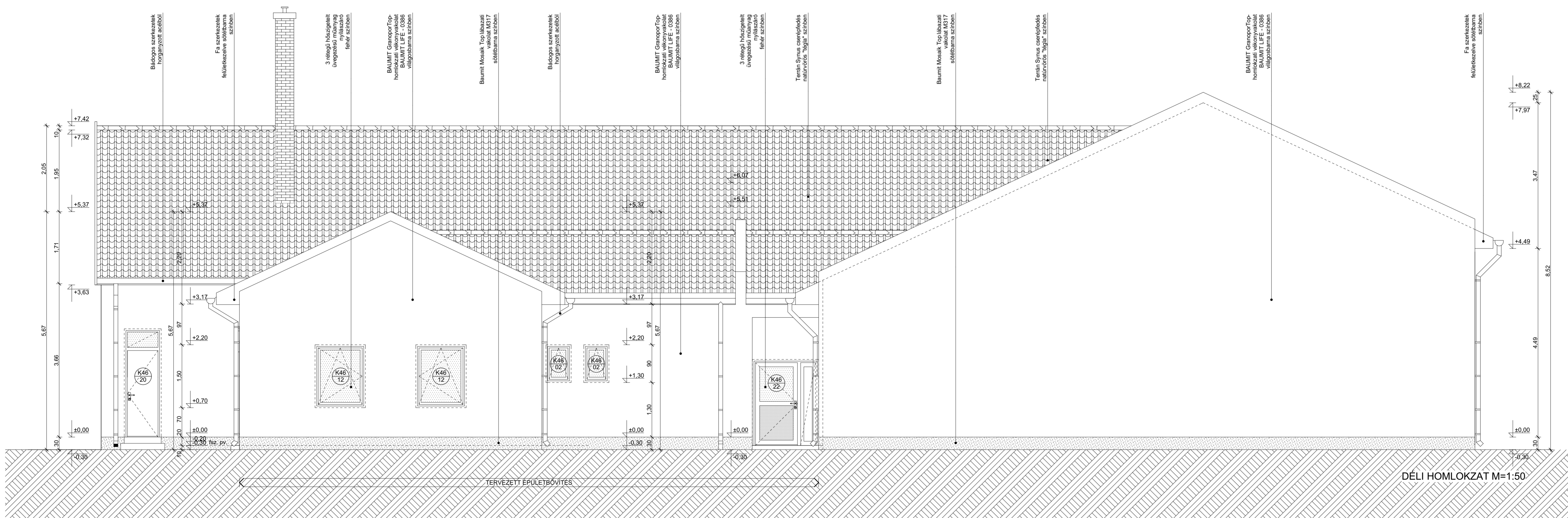
ÉSZAKI HOMLOKZAT M=1:50
